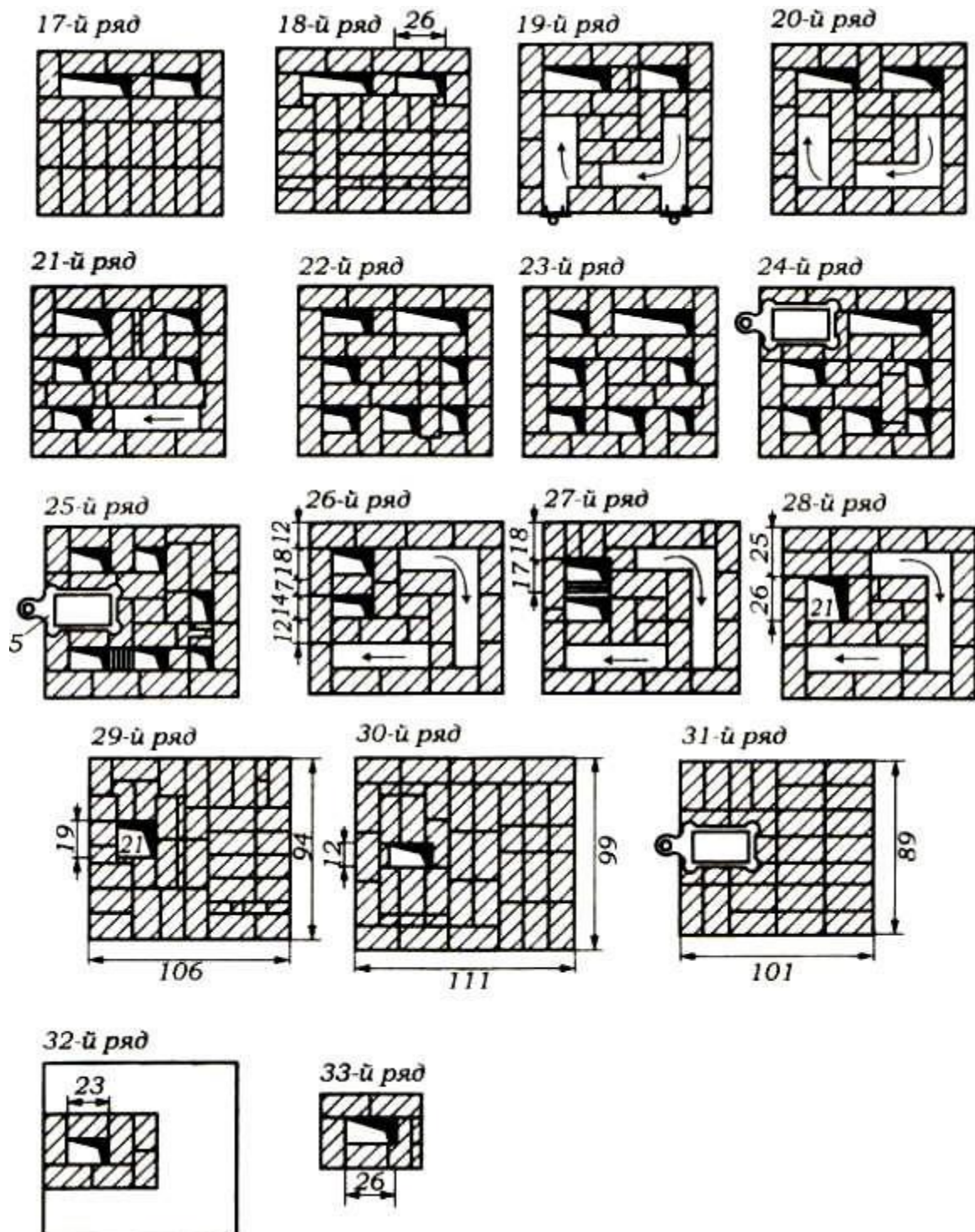
Рис. 2 Порядовка (размеры в см):
